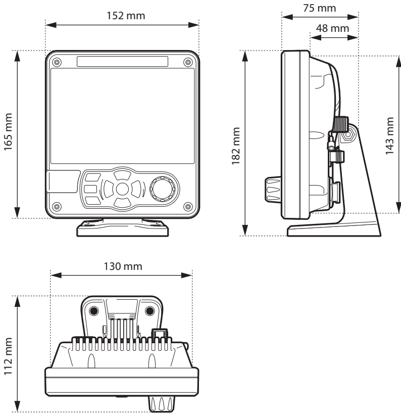
Afbeelding 30 Afmetingen van AIS-transponder
