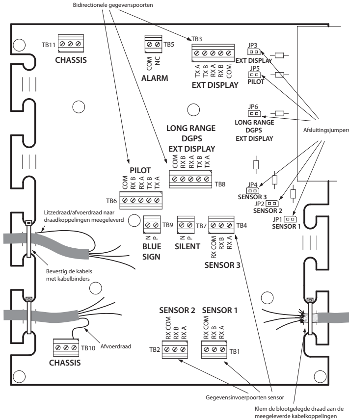
Afbeelding 33 Aansluitingen aansluitkast
