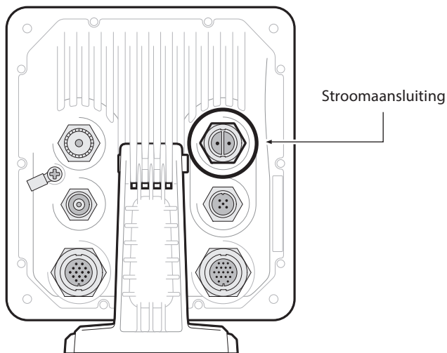
Afbeelding 15 Stroomaansluiting
