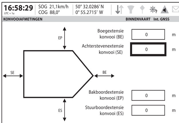
Afbeelding 26 Scherm Konvoiafmetingen
