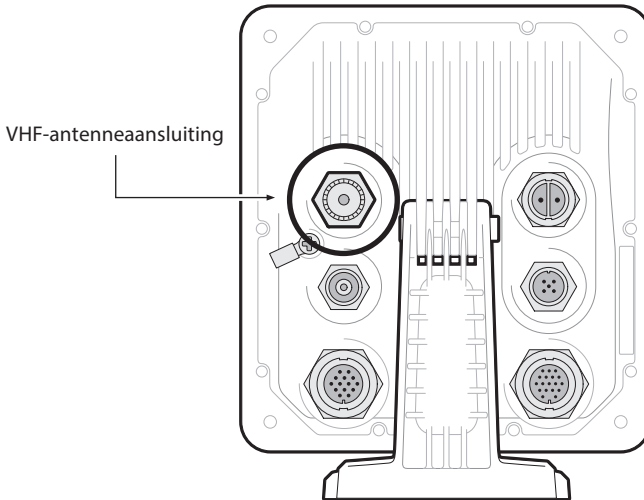
Afbeelding 10 Aansluiting VHF-antenne
