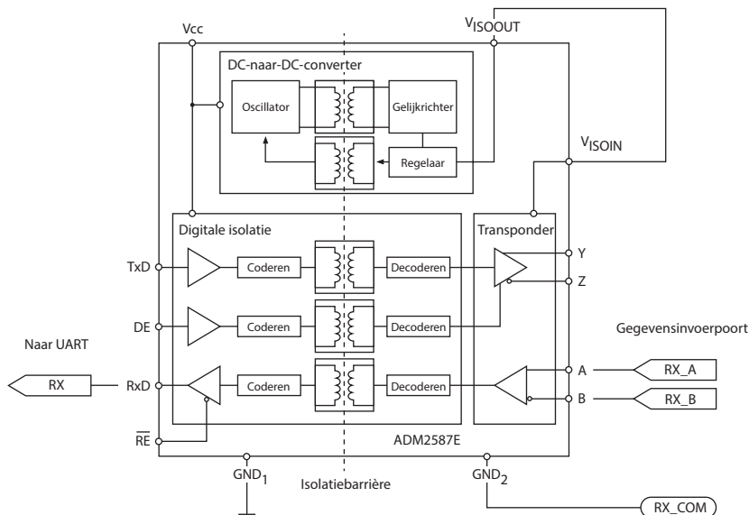
Afbeelding 28 Schema ingangspoort
